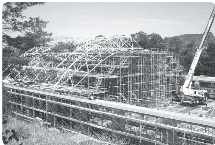
建築中のテニスコート上屋
