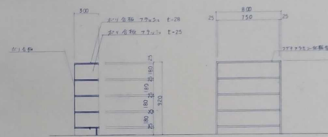
上足部収納詳細図 (作尺)
