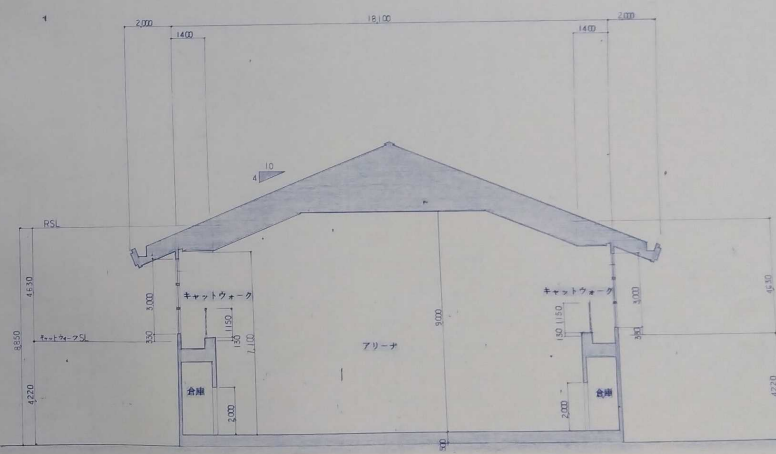
E-E 断面図
