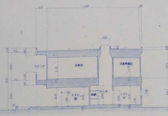
C-C 断面図
