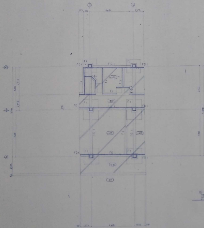
基礎位置
