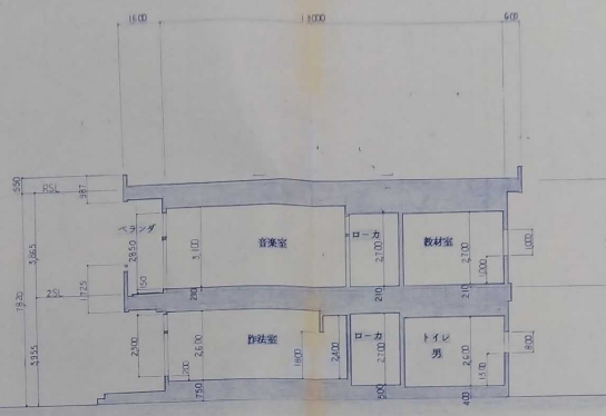
B-B 断面図
