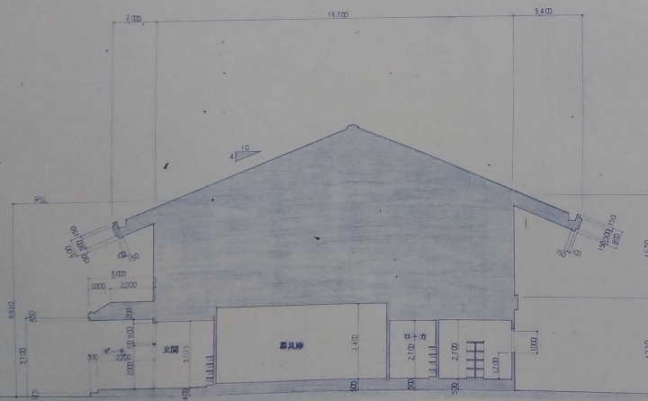
D-D 断面図
