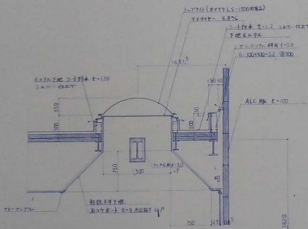
トップライト詳細図
