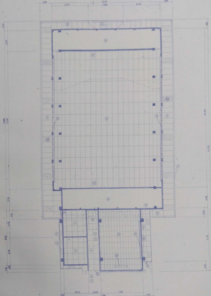
2階天井伏図
