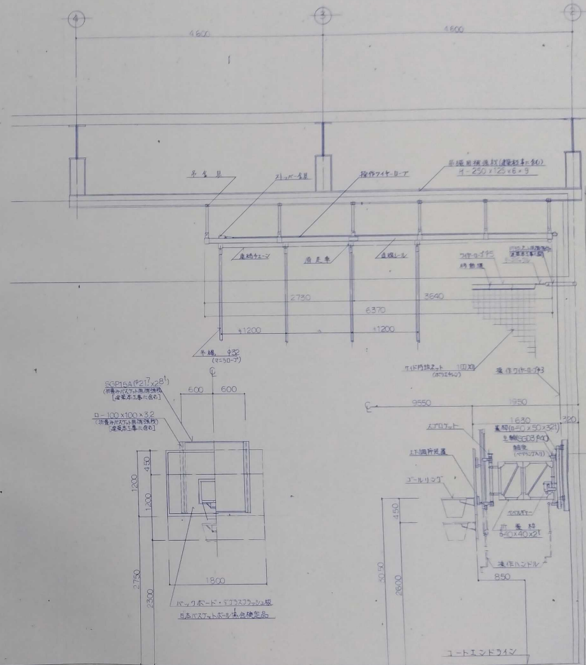
DC1106 壁面固定 折畳みハンド操作式バスケット板面 (日本バスケットボール協会規定品)
